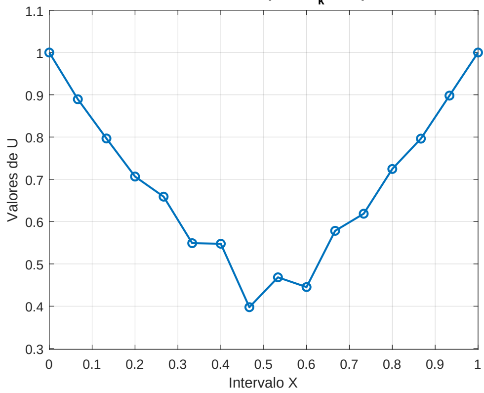
Iteración: 1000 ( n=15 , t_k=0.15 )
